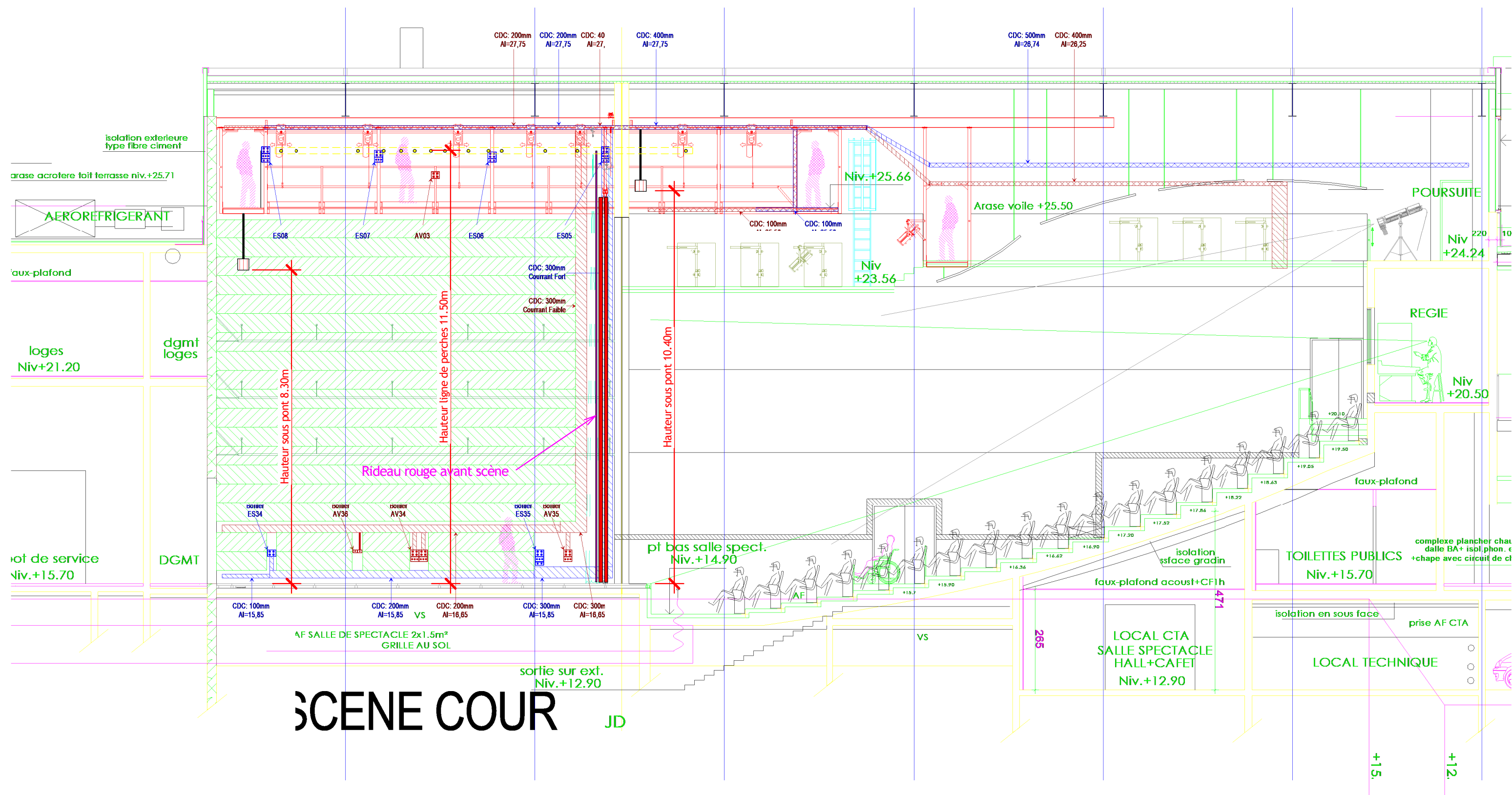
N COUPE 1 ET COUPE 7
